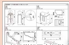
部品詳細図出力例
